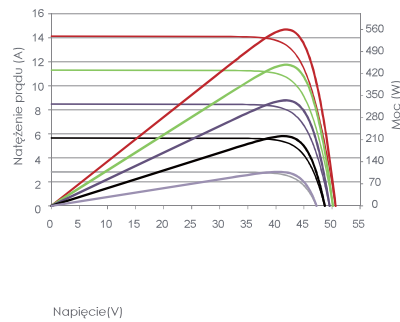
Krzywe prądowo-napięciowe i mocowo napięciowe (560 W)
